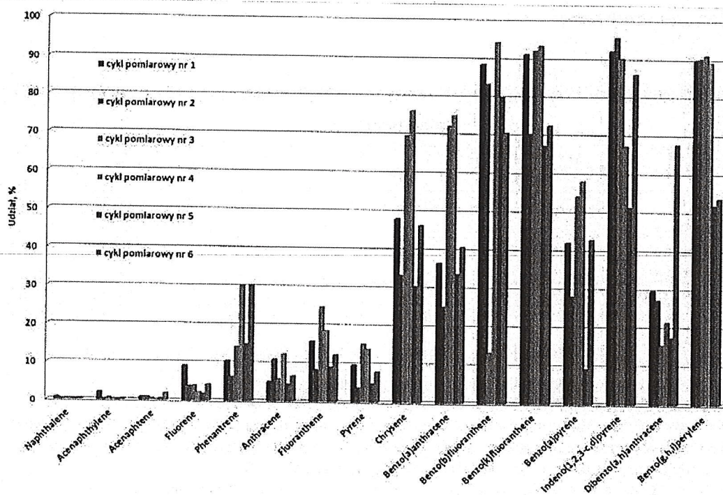
Rysunek 6.5. Oznaczony udział stężeń poszczególnych WWA w \mu\text{g}/\text{m}^3 w pyle, w stosunku do całkowitej emisji stężenia poszczególnych WWA ze spalania drewna w cyklach pomiarowych 1-6.
